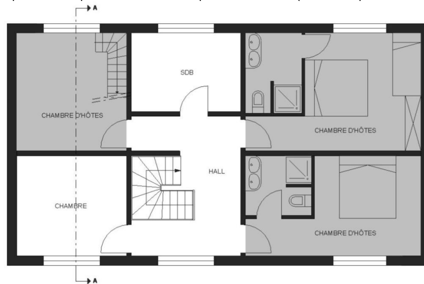
ETAGE
