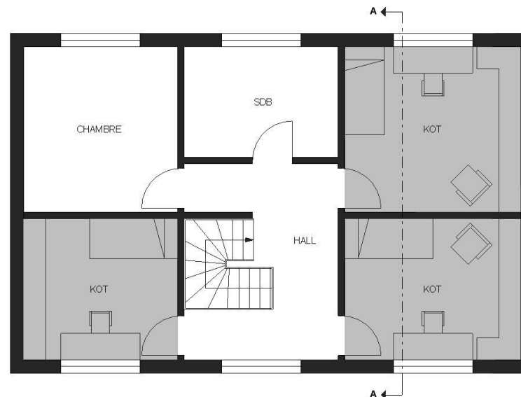
ETAGE
