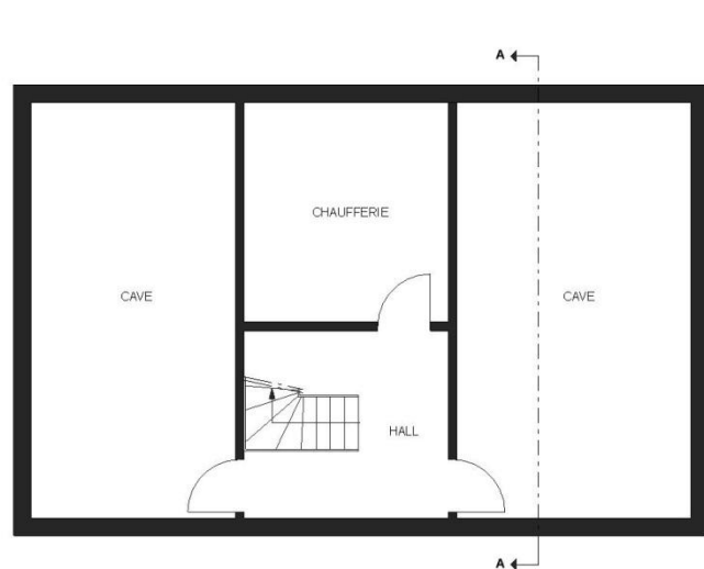
SOUS-SOL
