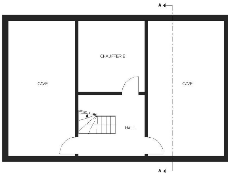
SOUS-SOL
