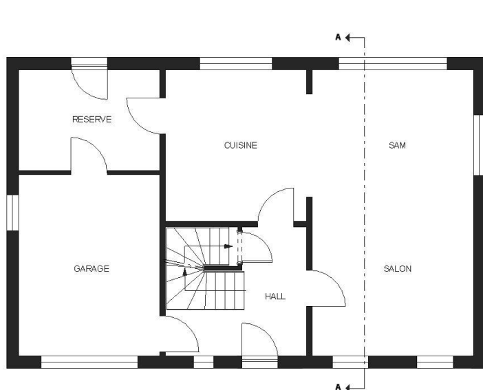
REZ-DE-CHAUSSEE
