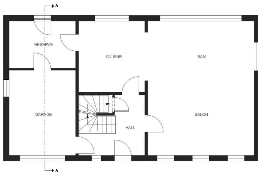
REZ-DE-CHAUSSEE
