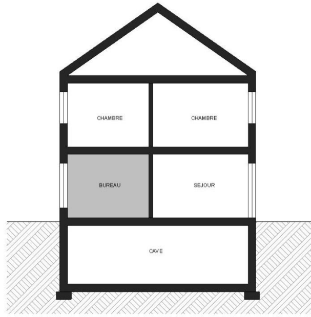
COUPE
