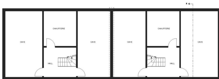
SOUS-SOL
