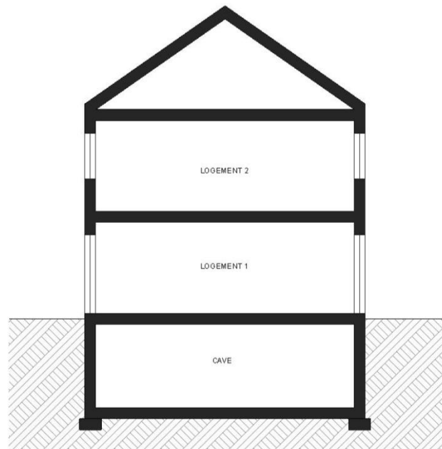
COUPE
